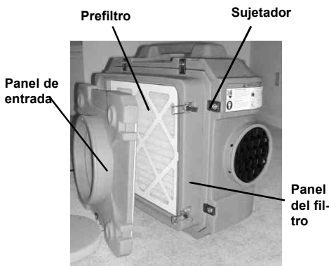
FIGURA 3 Prefiltro
