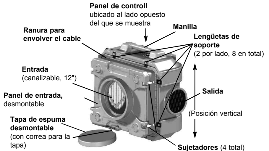
FIGURA 1 HEPA 500
